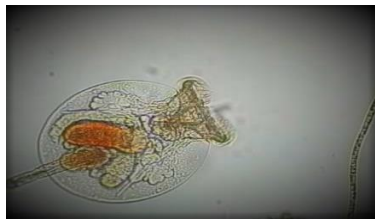
Testudinella sp.
