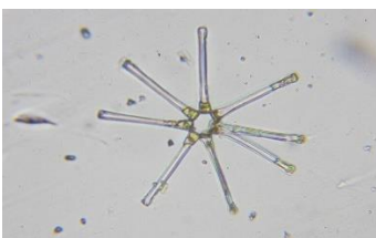
Asterionella sp.
